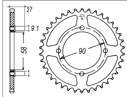
JTR 267
