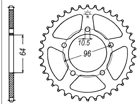
JTR 254
