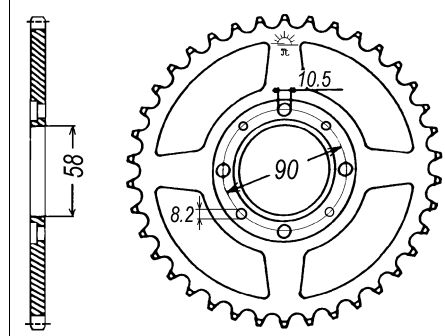
JTR 269
