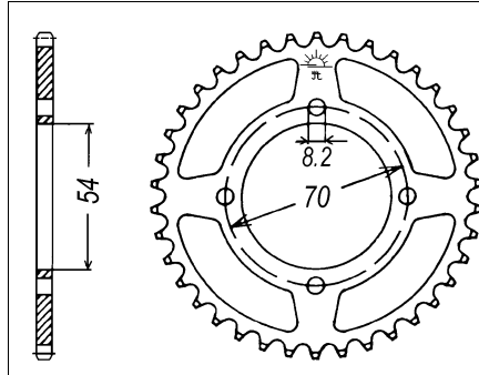
JTR 257
