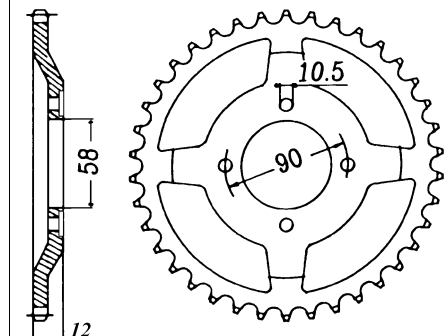
JTR 271
