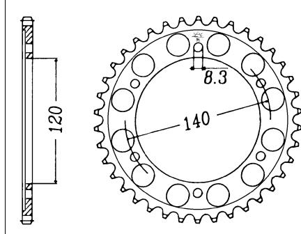
JTR 260
