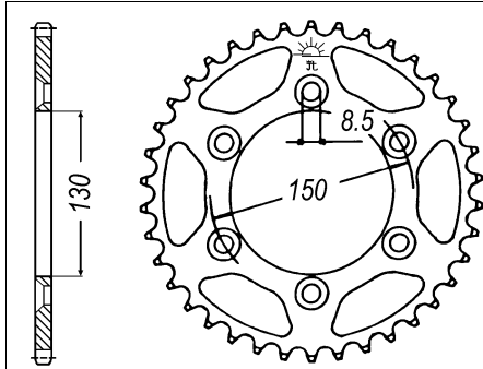
JTR 251
